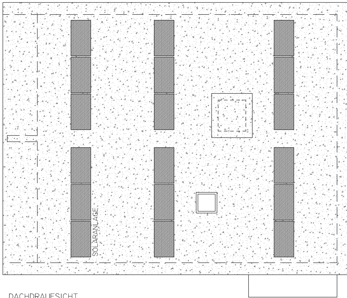
DACHDRAUFSICHT M I-100
